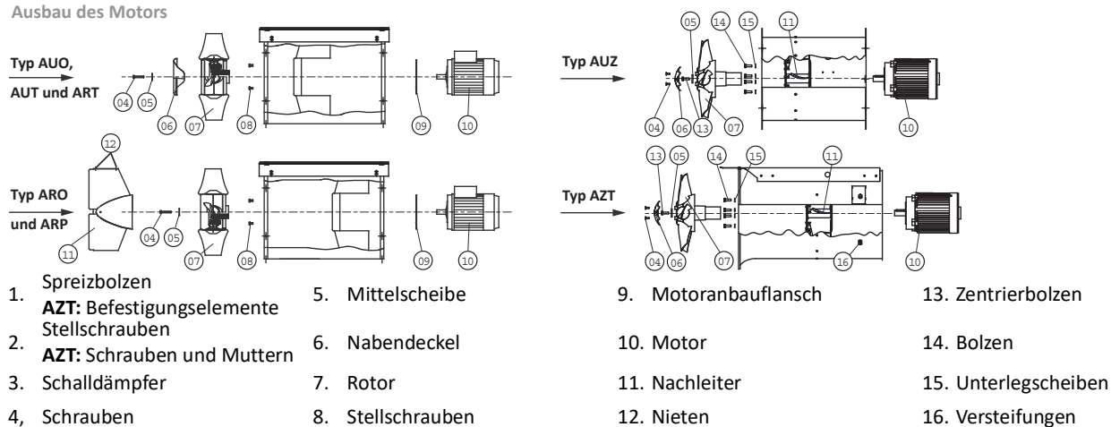
Abbildung 8. Hauptkomponenten
