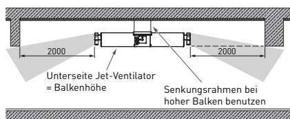
Abbildung 2. Mindestabstandsanforderungen für umkehrbare Jet-Ventilatoren
